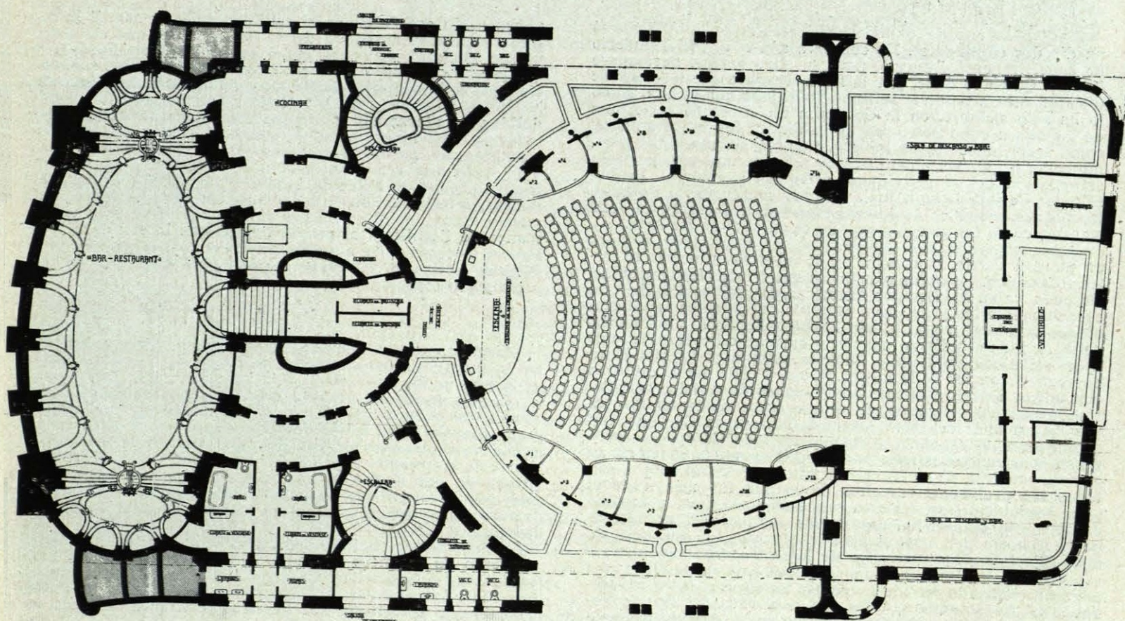
Planta del patio de butacas.
